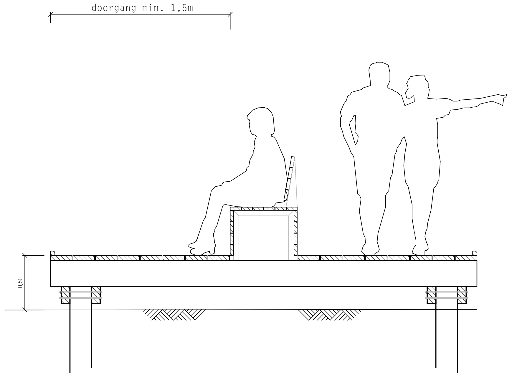
Principeprofiel eiland
