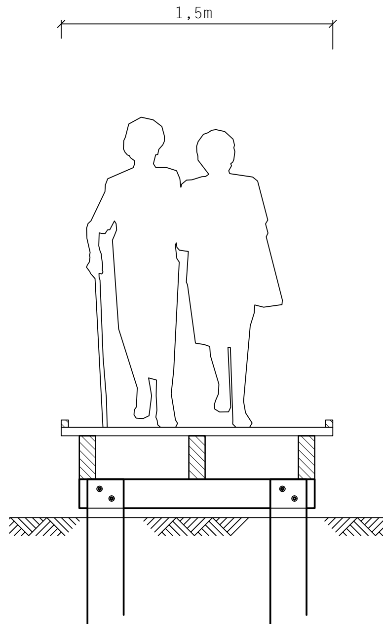
Principeprofiel looppad
