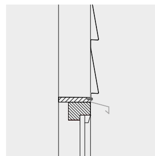
lekdorpeldetail
