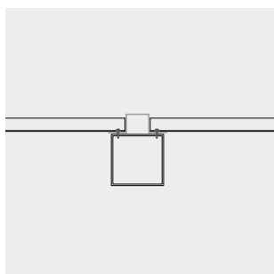
stuikdetail
